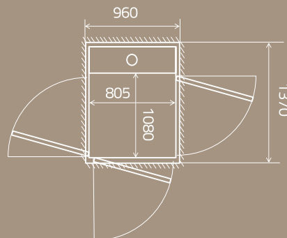
Taille: 1080 x 805 mm Charge nominale: 250 kg / 2 personnes
