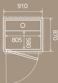
Taille: 580 x 805 mm Charge nominale: 250 kg / 2 personnes
